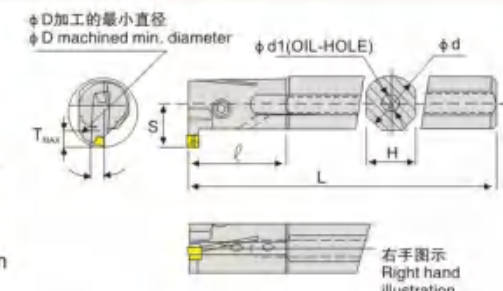
进给方向 Feed direction
